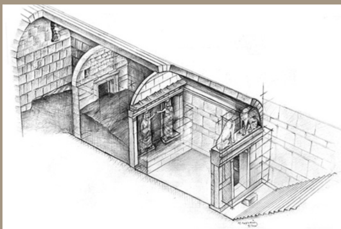
Εικ. 3. Αξονομετρική τομή ταφικού μνημείου
