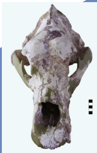
Εικ 6. Κρανίο αρκούδας, από το δάπεδο του σπηλαίου (Φωτογραφικό αρχείο ΕΠΣ).
