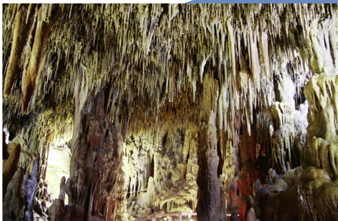
Εικ 2. Άποψη αίθουσας του σπηλαίου κατάκοσμη με σταλαγμιτικούς σχηματισμούς (Φωτογραφικό Αρχείο ΕΠΣ).
