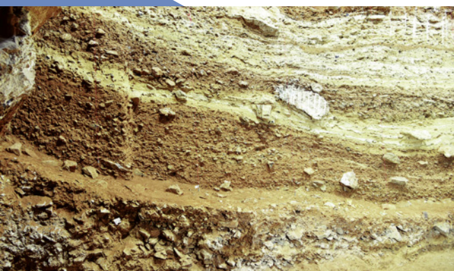
Εικ 4. Μερική άποψη της ανασκαφικής παρείας. Διακρίνονται τα διαδοχικά στρώματα με τα κατάλοιπα που περιέχουν. Στο κάτω μέρος της εικόνας διακρίνονται τα πυκνά κατάλοιπα (οστά και λίθινα εργαλεία) μιας ανθρώπινης εγκατάστασης που αποκαλύπτει η ανασκαφή (Φωτογραφικό αρχείο ΕΠΣ).
