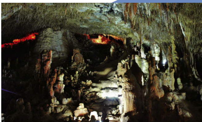
Εικ 3. Άποψη της πλευράς του κώνου κορημάτων που έχει σχηματιστεί κάτω από την αρχική είσοδο του σπηλαίου, στην επιφάνεια του οποίου έχουν αναπτυχθεί πυκνοί και μεγάλοι σταλαγμίτες (Φωτογραφικό Αρχείο ΕΠΣ).
