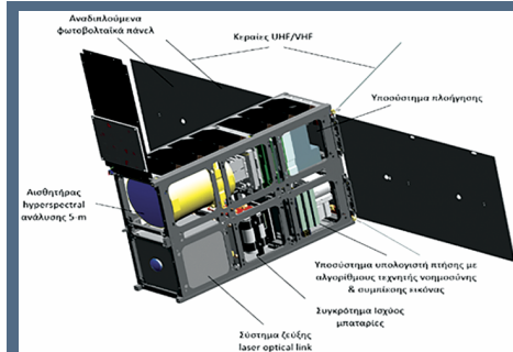
Εικόνα 9: Σχέδιο του νανο-δορυφόρου του προγράμματος «ΕΡΜΗΣ» που προορίζεται για γεωπαρατήρηση 33
