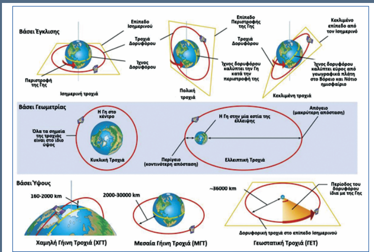
Εικόνα 1: Γήινες τροχιές δορυφόρων 4
