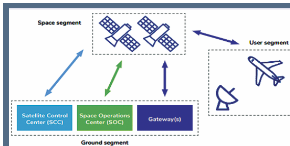
Εικόνα 2: Γενικό διάγραμμα ροής δορυφορικών τηλεπικοινωνιών 5
